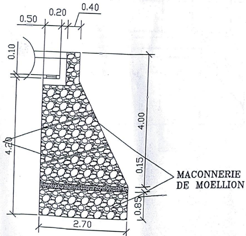
COUPE DE LA CULEE
